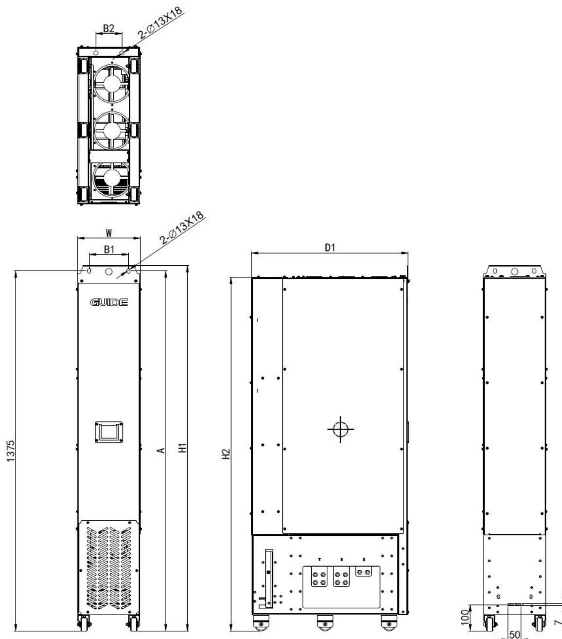
B7 机型 LCL 滤波单元外形示意图
