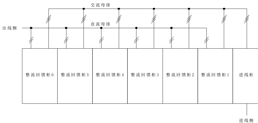
12脉并机示例 1
