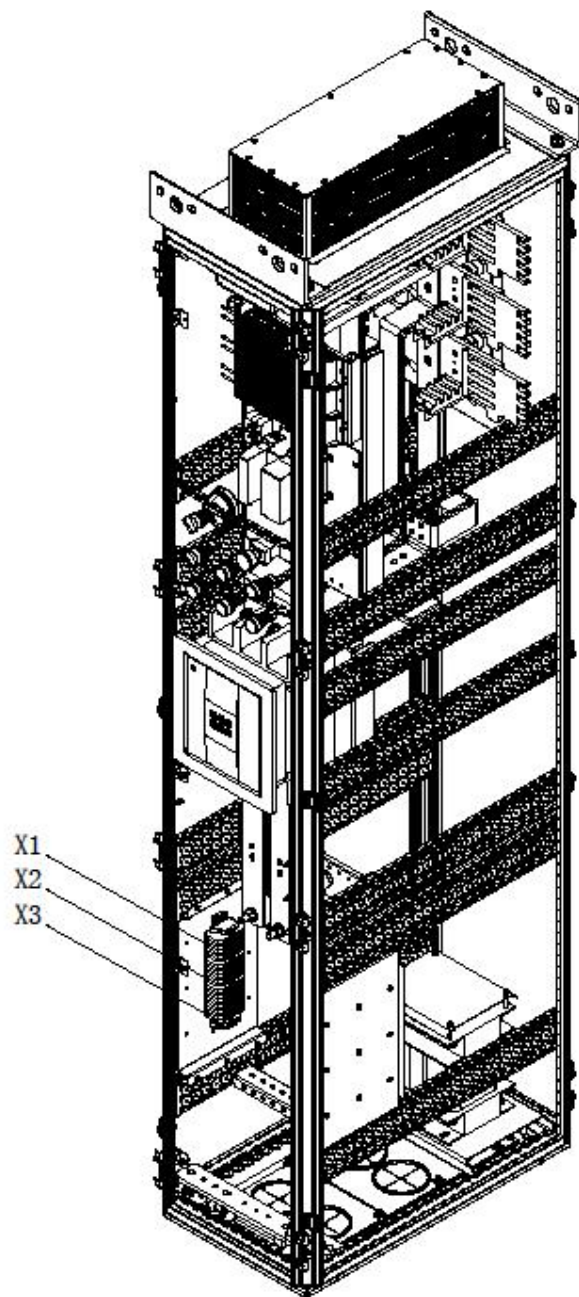
进线标准成柜接线端子位置示意图 (a)
