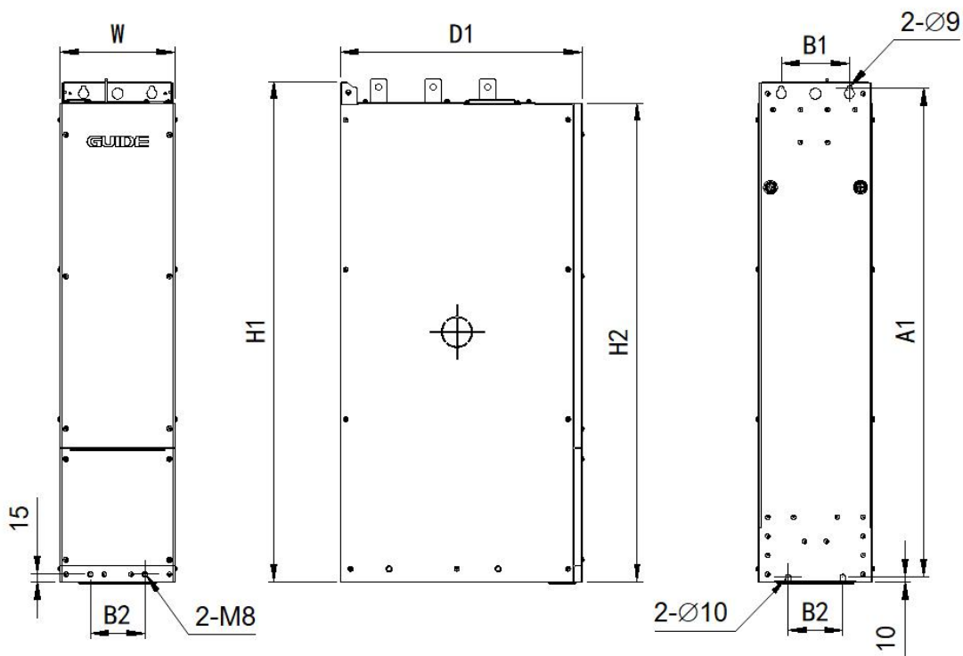
132kW LCL 滤波单元外形示意图
