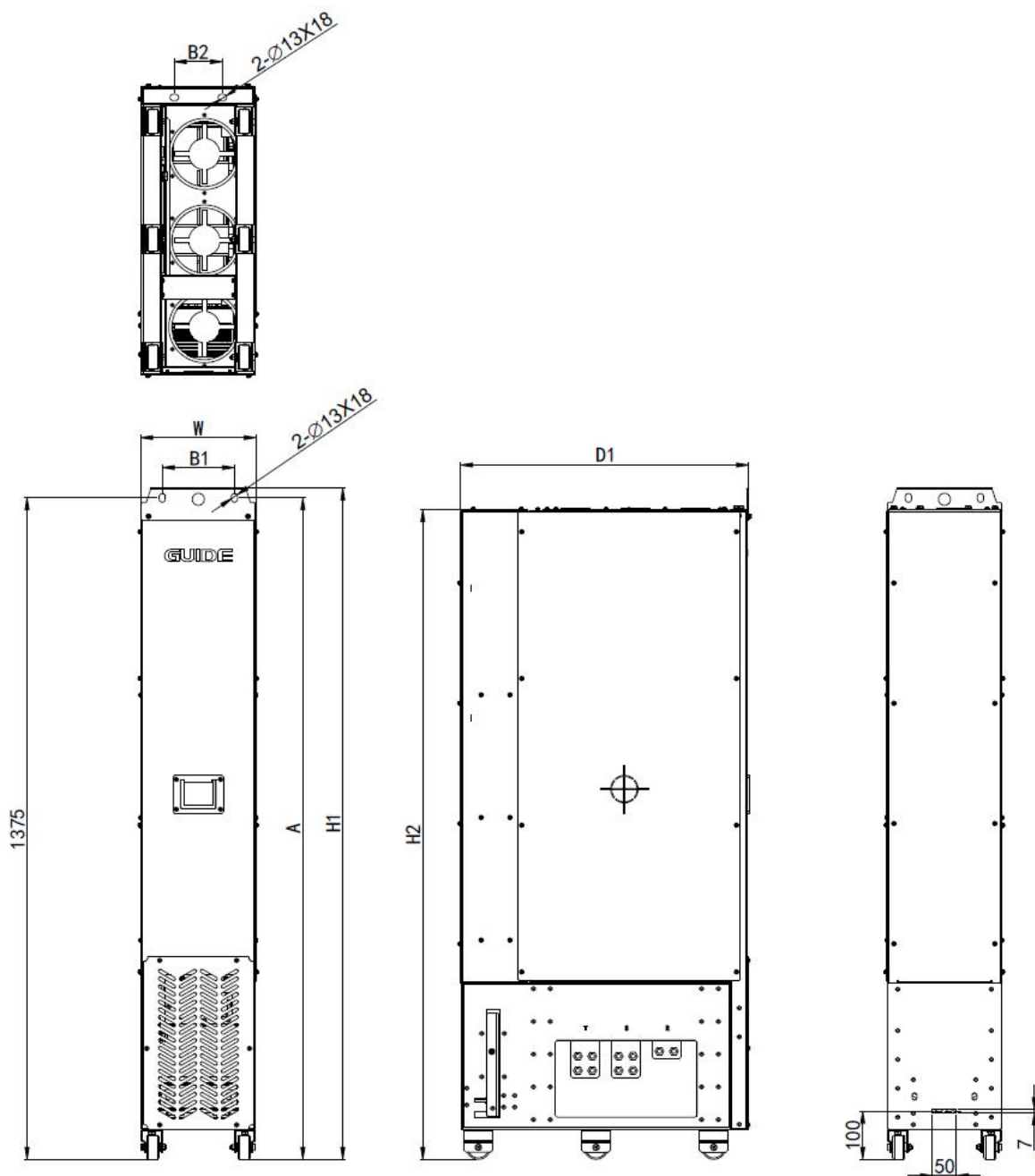
B7 机型 L 滤波单元外形示意图
