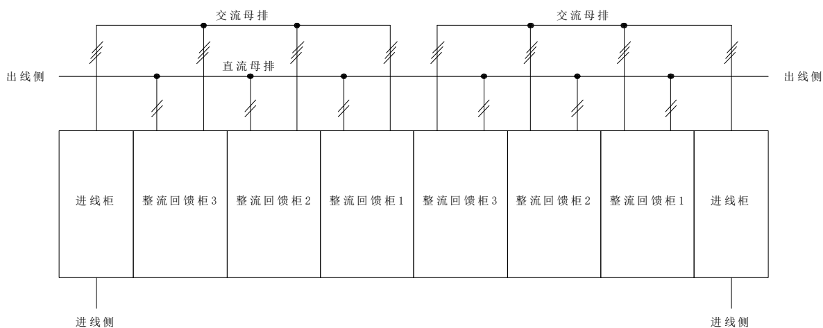
12脉并机示例 2
