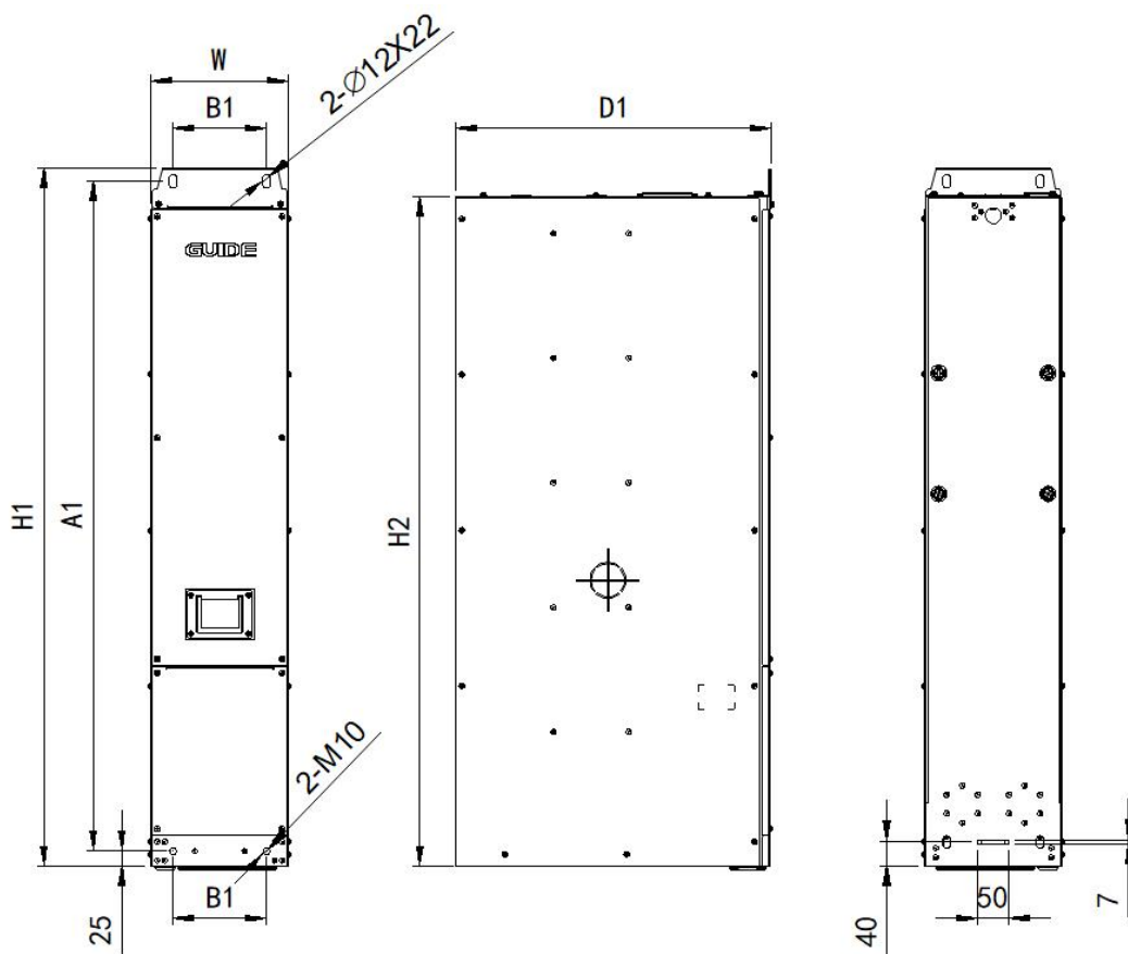
185kW LCL 滤波单元外形示意图
