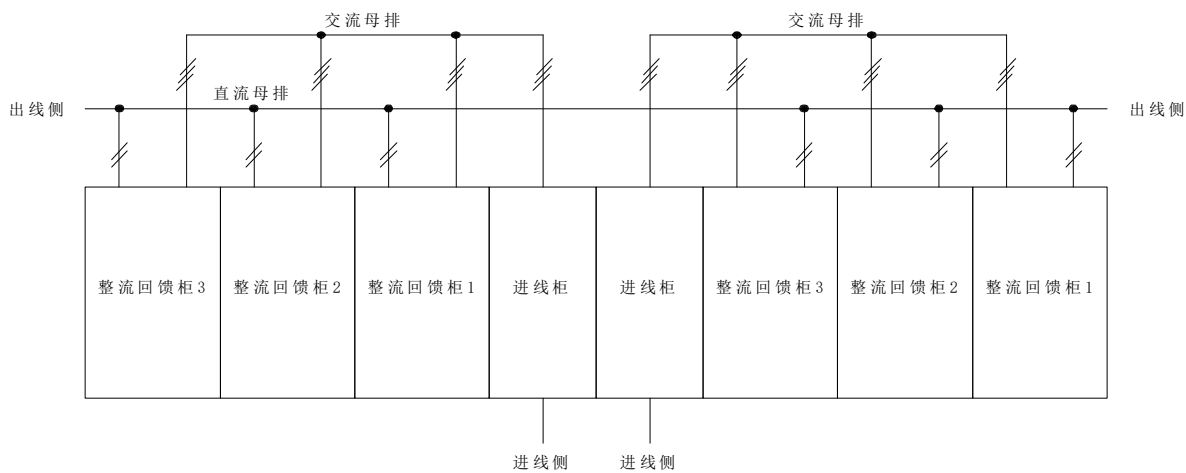
12脉并机示例 1
