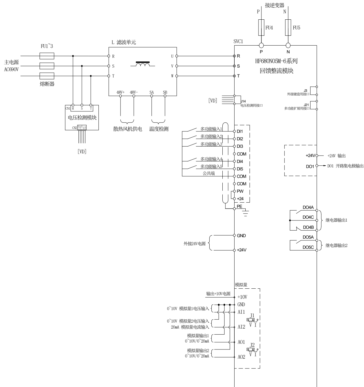
回馈整流单元的单机主回路图：
