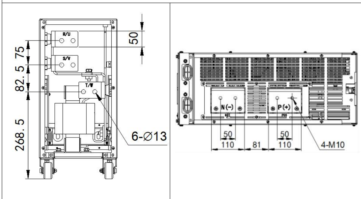
B7主回路端子分布图
