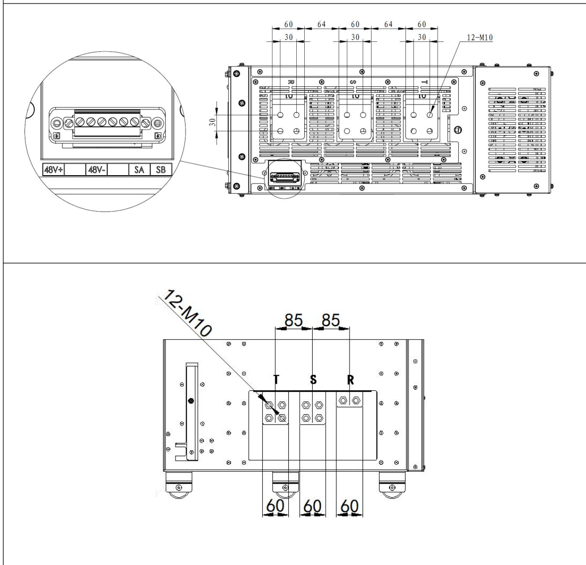
B7机型LCL端子分布图
