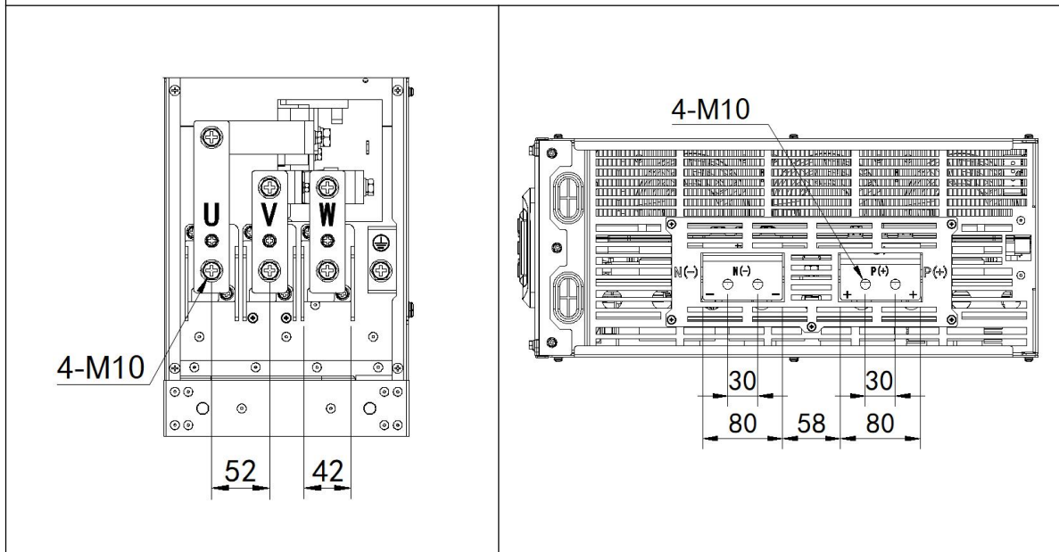
B7主回路端子分布图
