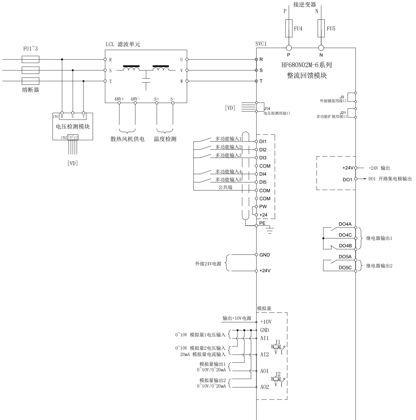
整流回馈单元的单机主回路图：
