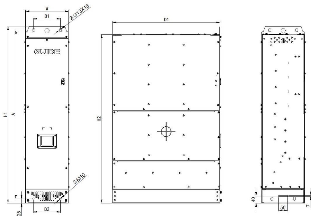
B7A 外形示意图
